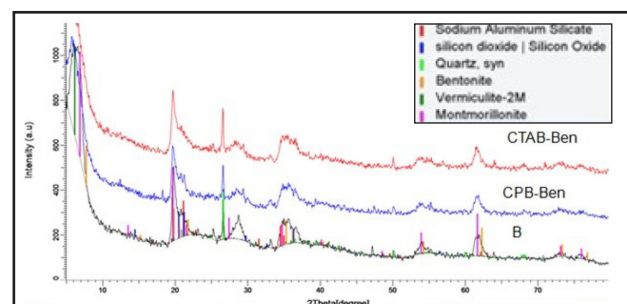
Figure 3: XRD patterns of NB, CPB-Ben and CTAB-Ben.
