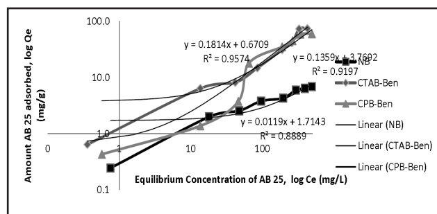
Figure 10: Freundlich isotherm graph for NB, CTAB-Ben and CPB-Ben.
